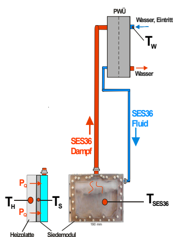
PWÜ: Plattenwärmeübertrager
