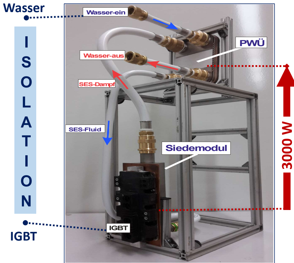
PWÜ: Plattenwärmeübertrager
